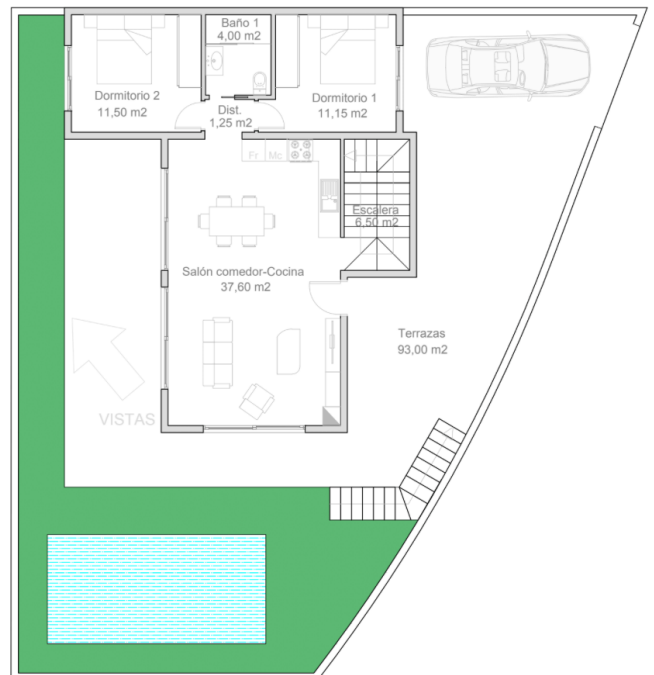
PLANTA INTERMEDIA
