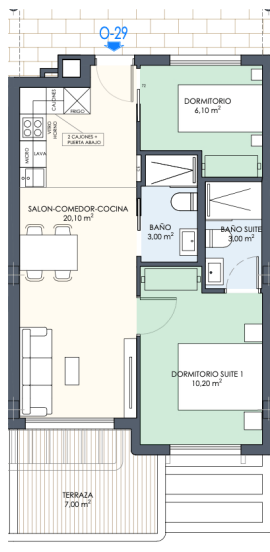
PLANTA PRIMERA
