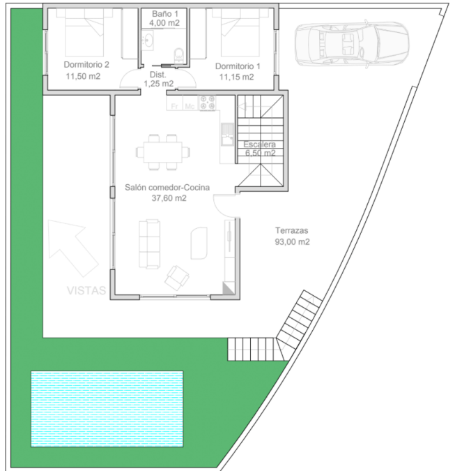
PLANTA INTERMEDIA
