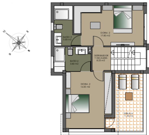
PLANTA PISO
