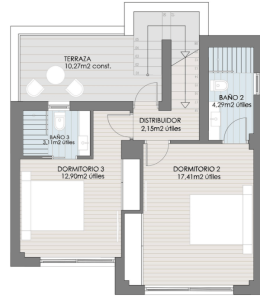
PLANTA PRIMERA E: 1/75
