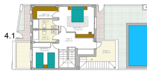
Planta Primera
