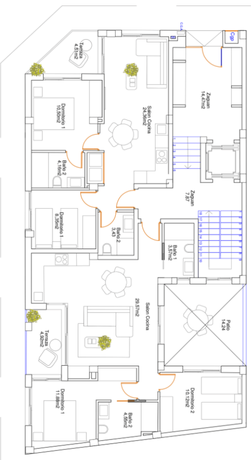
PLANTA BAJA.
