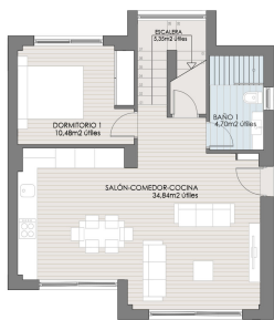
PLANTA BAJA E: 1/75
