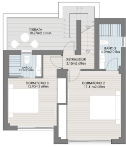
PLANTA PRIMERA E: 1/75
