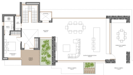
PLANTA BAJA
