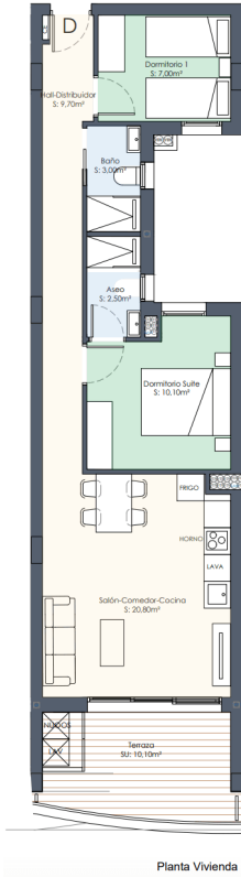
Planta Vivienda
