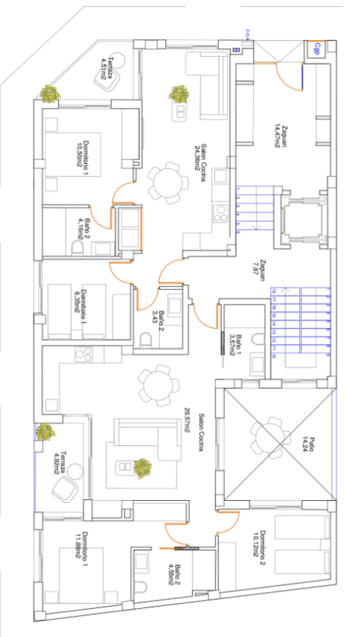
PLANTA BAJA.
