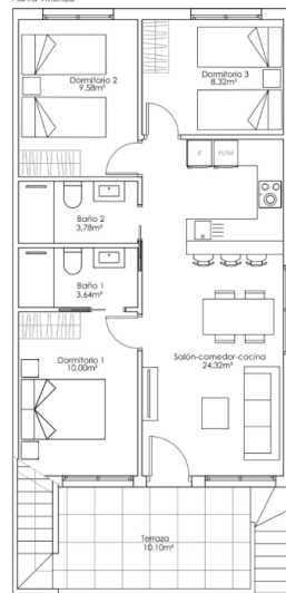
Planta Vivienda
