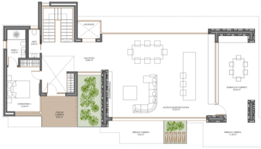
PLANTA BAJA
