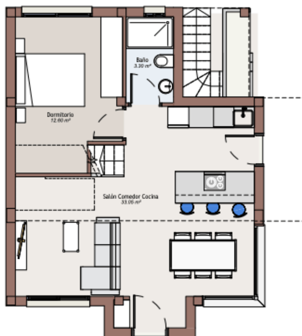
PLANTA 1 - BAJA
