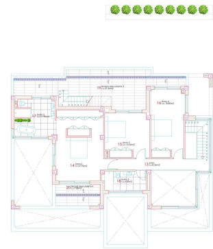
PLANTA PRIMERA
