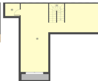
PLANTA SÓTANO
