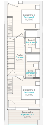
Planta Alta | Top Floor
