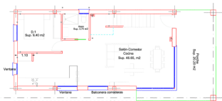
Planta Baja
