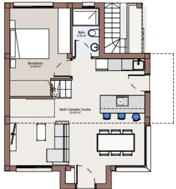
PLANTA 1 - BAJA
