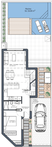
PLANTA BAJA
