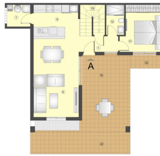
PLANTA BAJA
