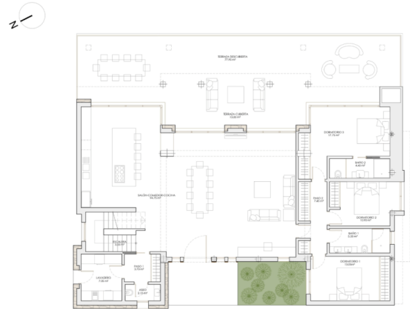
PLANTA NIVEL 0
