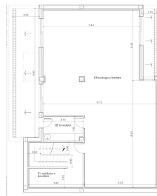
Planta sótano COTAS Y CUMPLIMIENTO DC-09
