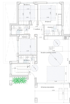
Planta baja COTAS Y CUMPLIMIENTO DC-09
