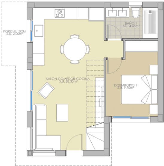
PLANTA BAJA OPCIÓN 1
