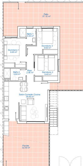
PLANTA BAJA
