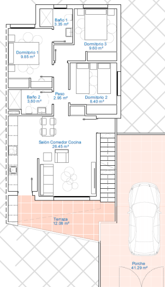
PLANTA PRIMERA
