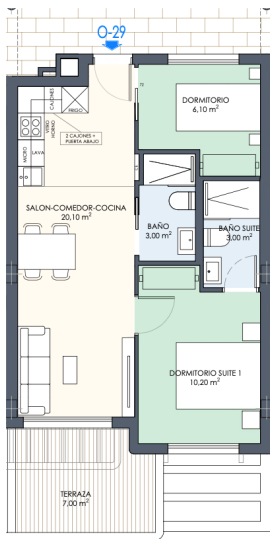
PLANTA PRIMERA
