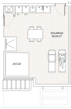
PLANTA SOLARIUM
