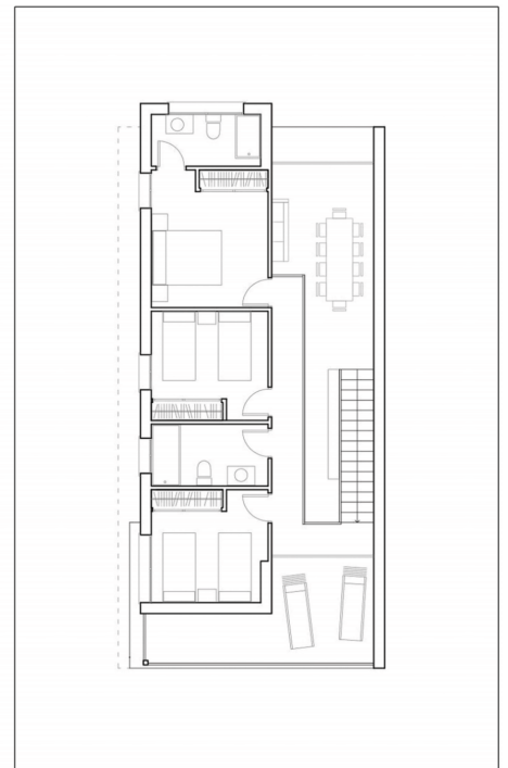
PLANTA PRIMERA
