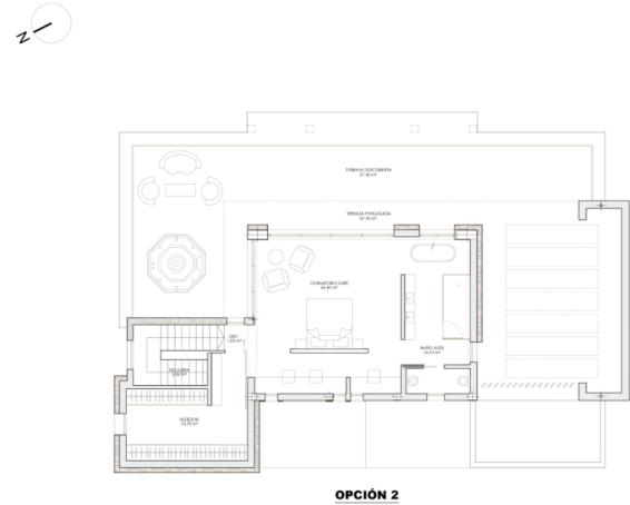
PLANTA NIVEL +1
