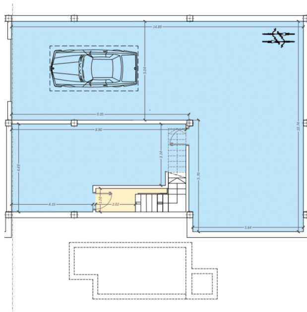
PLANTA SOTANO
