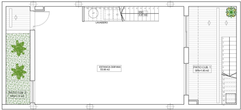
PLANTA SÓTANO
