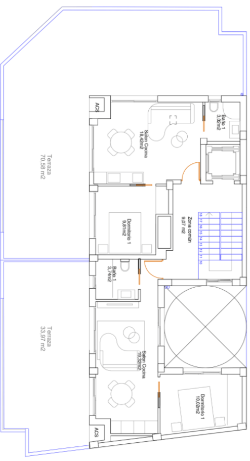
PLANTA ÁTICO.
