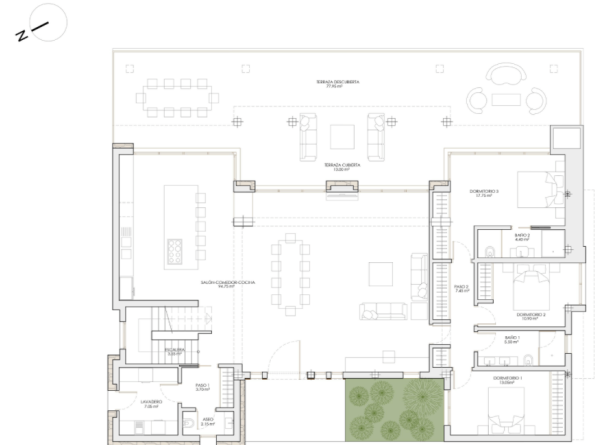
PLANTA NIVEL 0
