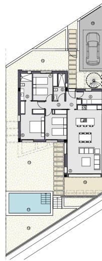
PLANTA BAJA
