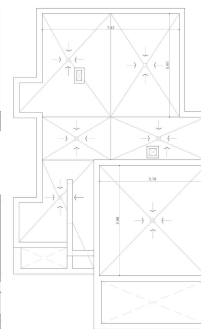
Planta cubierta COTAS
