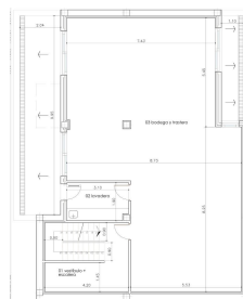
Planta sótano COTAS Y CUMPLIMIENTO DC-09
